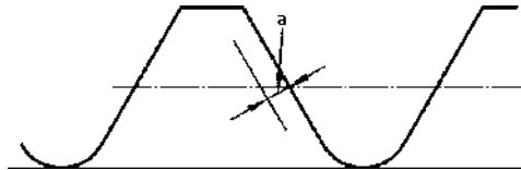
Bild 2 — Stelle, an der die Einsatzhärtungstiefe gemessen werden darf
