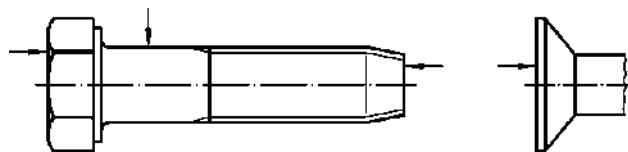
Bild 1 — Stellen, an denen die Oberflächenhärte gemessen werden darf
